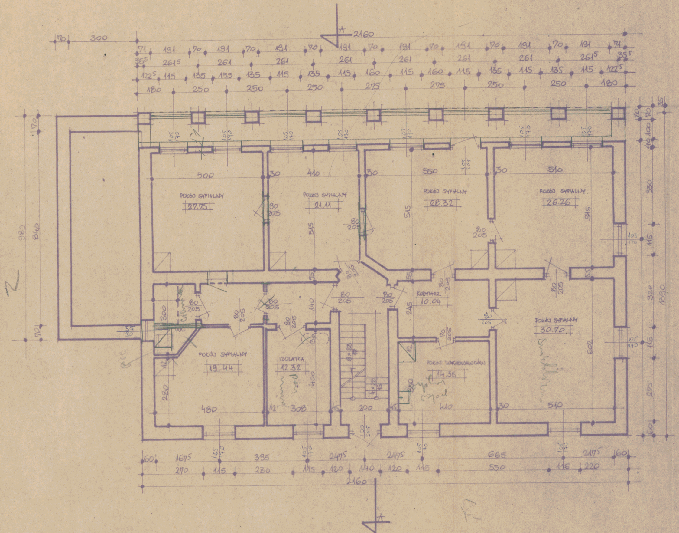
RZUT PARTERU SKALA 1:100
