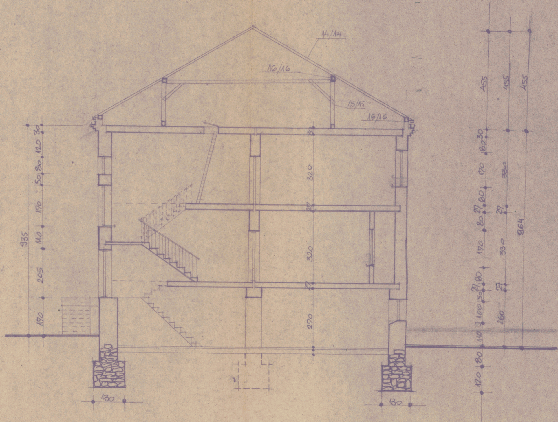
PRZEKROJ A-A SKALA 1:100
