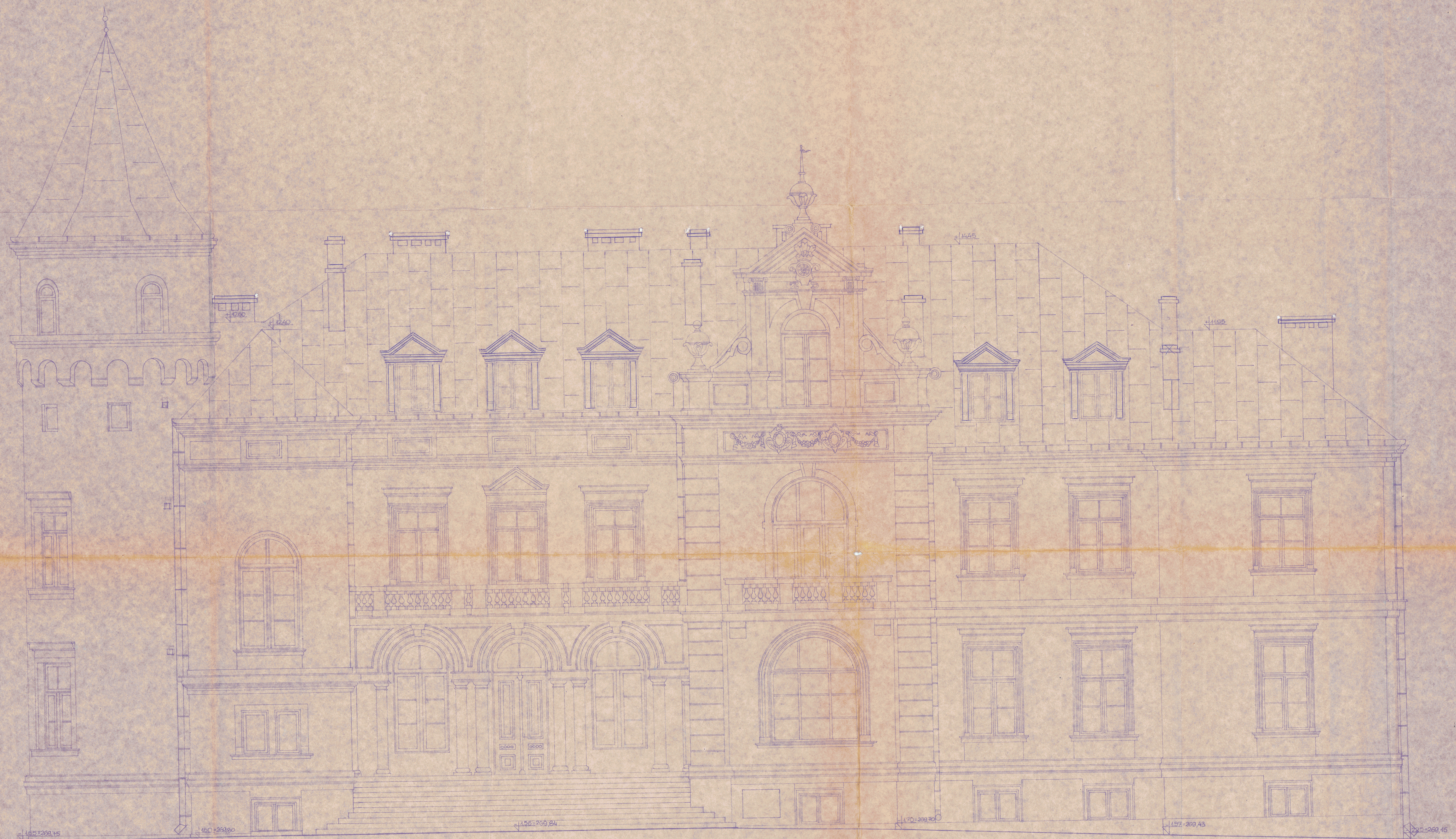
ELEWACJA PÓLNOČNA 1:50
