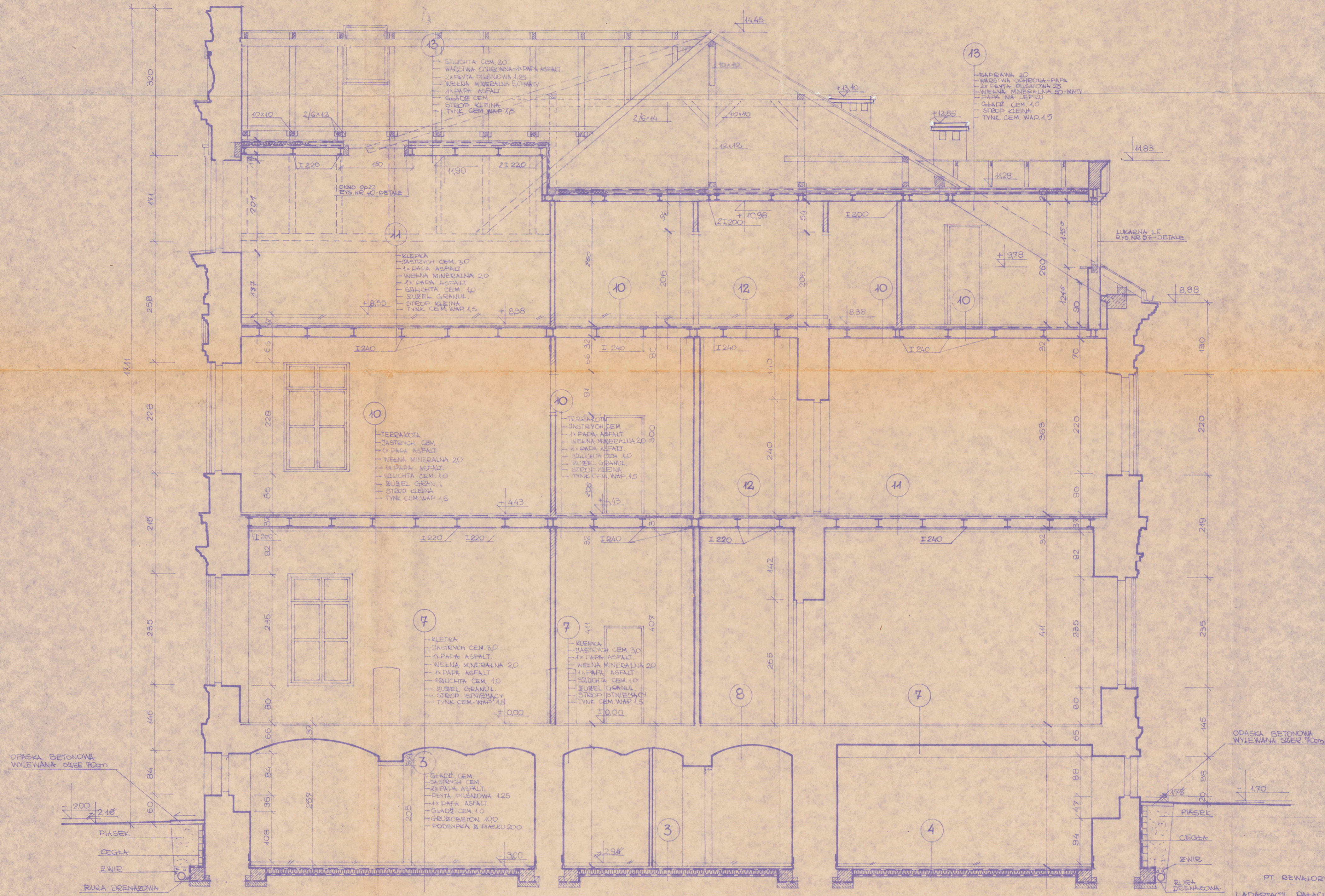
PRZEKRÓJ IV-IV SKALA 1:50
