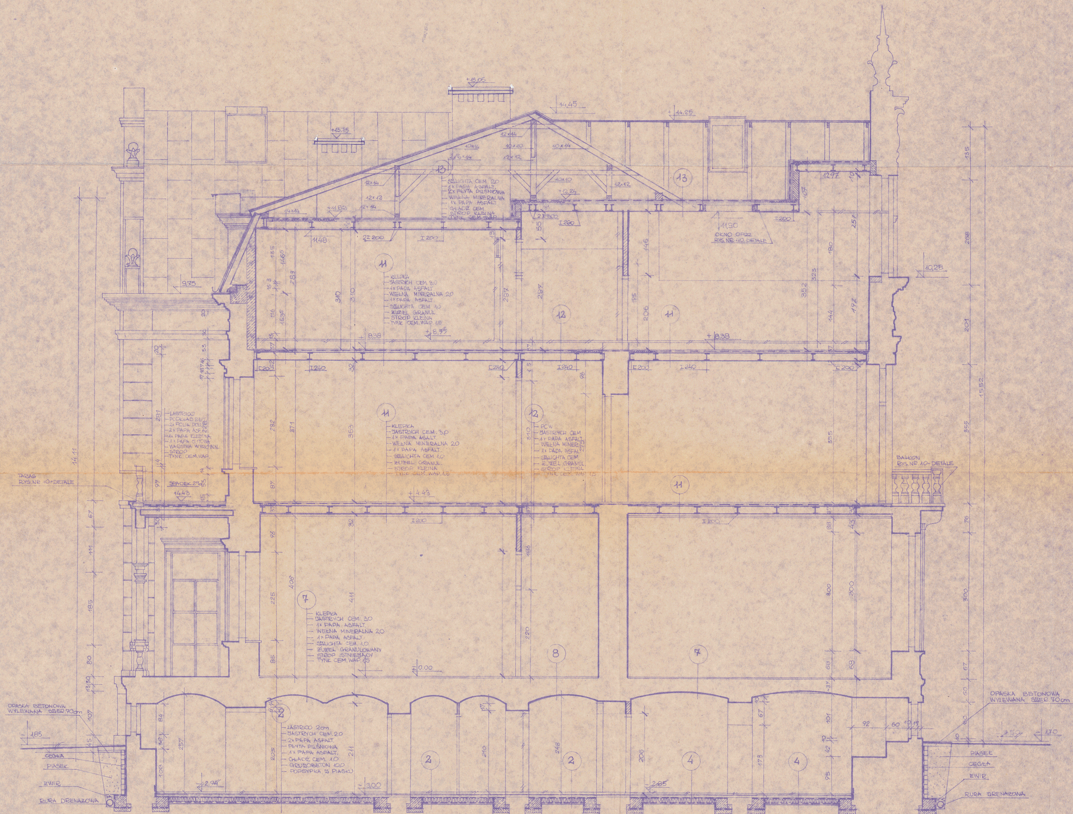
PRZEKRÓJ III-III. SKALA 1:50.
